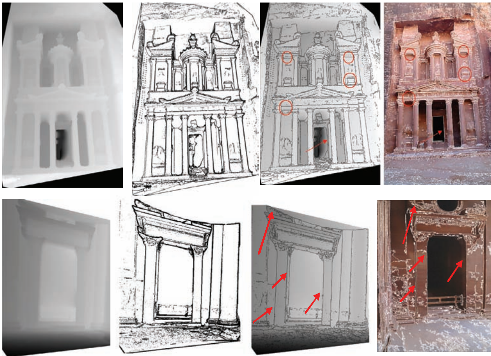
Abb. 4: a) Distanzbilder der Khazne al-Firaun, b) Segmentierte Bruchkanten im zugehörigen Distanzbild, c) Skelettierte Bruchkanten im zugehörigen Distanzbild, d) Segmentierung der Bilddaten. Für die Registrierung der Bild- und Distanzdaten ausgewählte Segmente sind durch Pfeile bzw. Kreise markiert.
