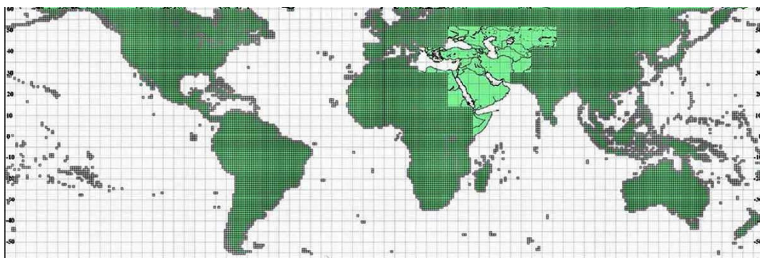
Abb. 2: dunkelgrün = am 22.9.2014 September freigegebene SRTM DOM mit 1 arcsec Punktabstand, hellgrün = Beschränkung auf 3 arcsec Punktabstand (USGS)
